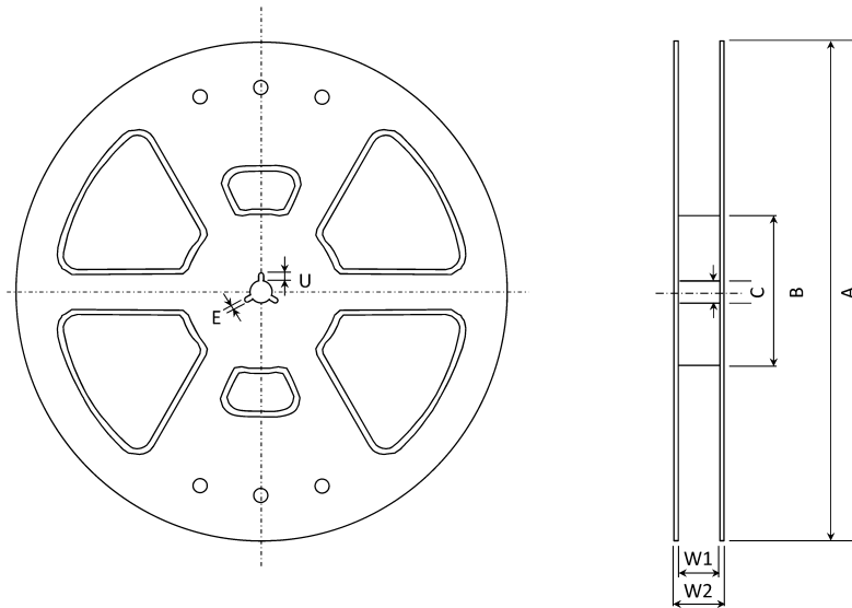
Fig. 16.3.5.1 Reel Dimensions
