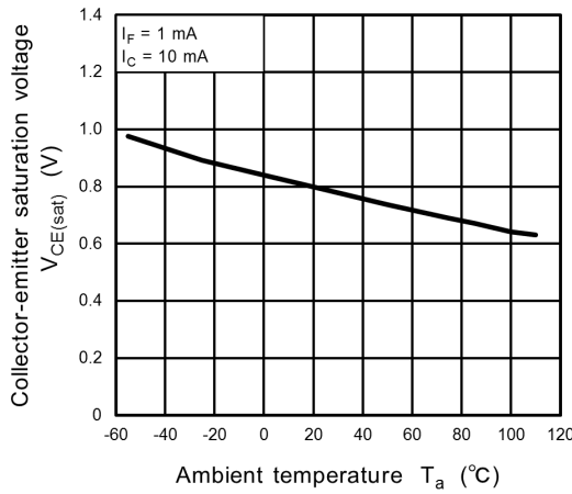
Fig. 11.9 V_{CE(sat)} - T_a
