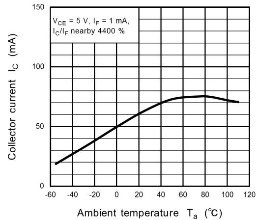
Fig. 11.12 I_C - T_a
